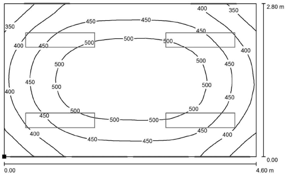
工作面 Work-Plane
